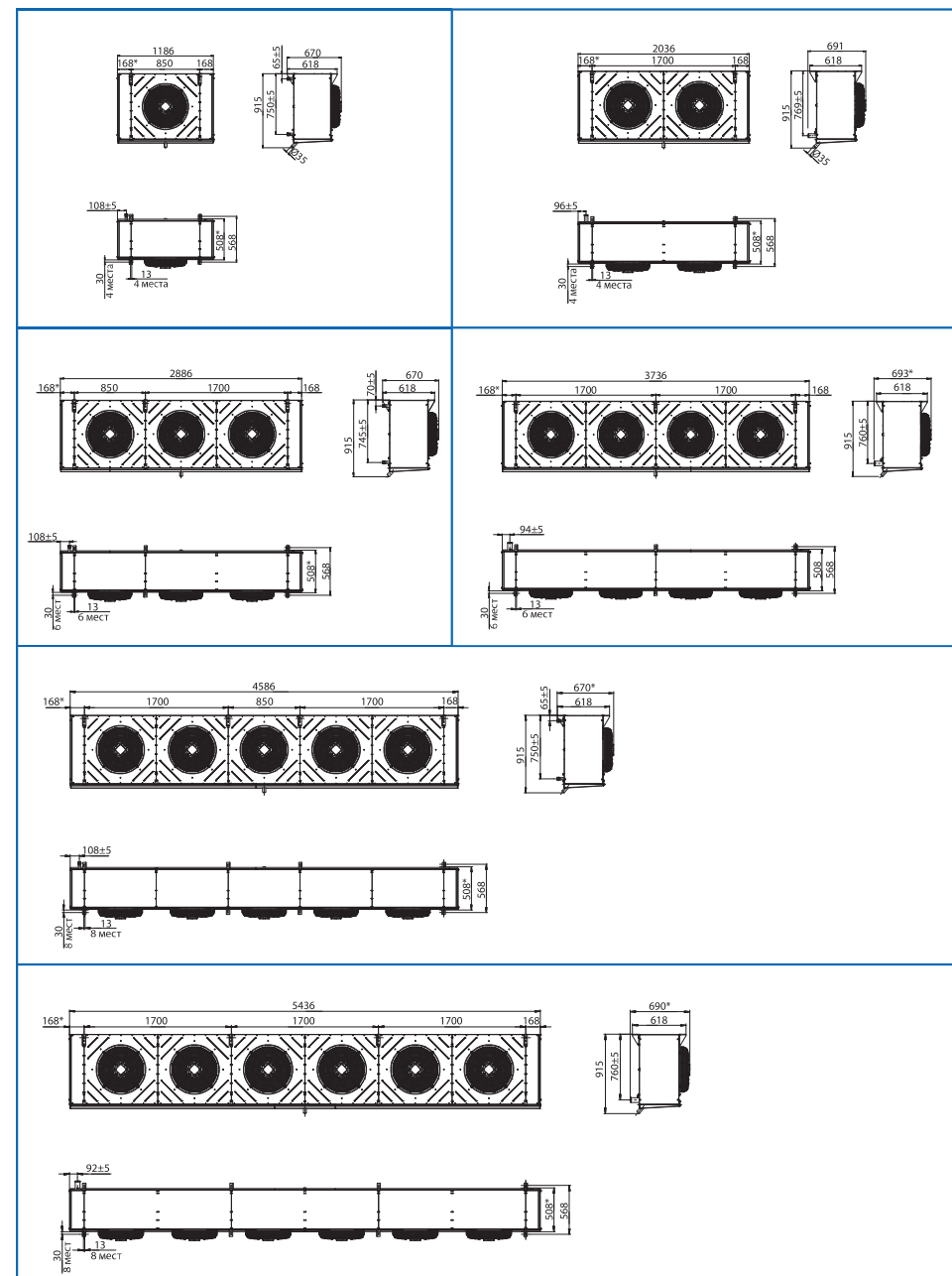
Габаритные и присоединительные размеры UCR.500
