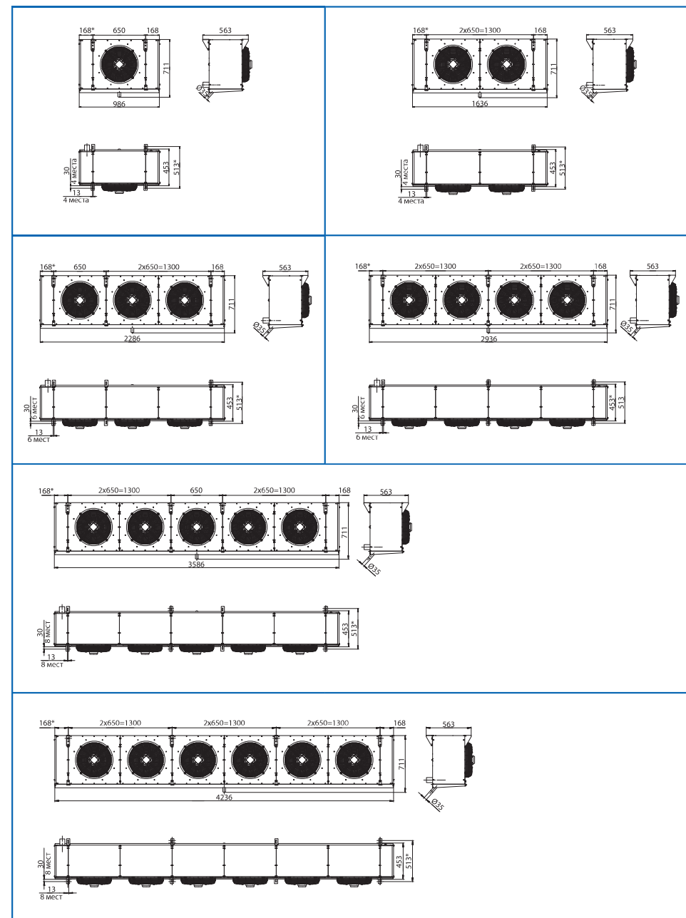
Габаритные и присоединительные размеры UCR.400
