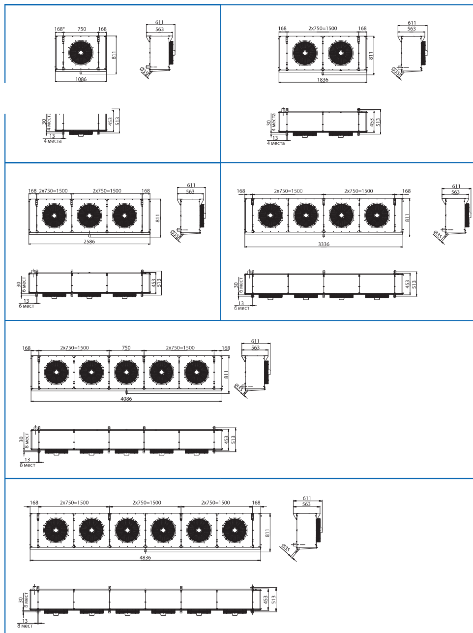
Габаритные и присоединительные размеры UCR.450
