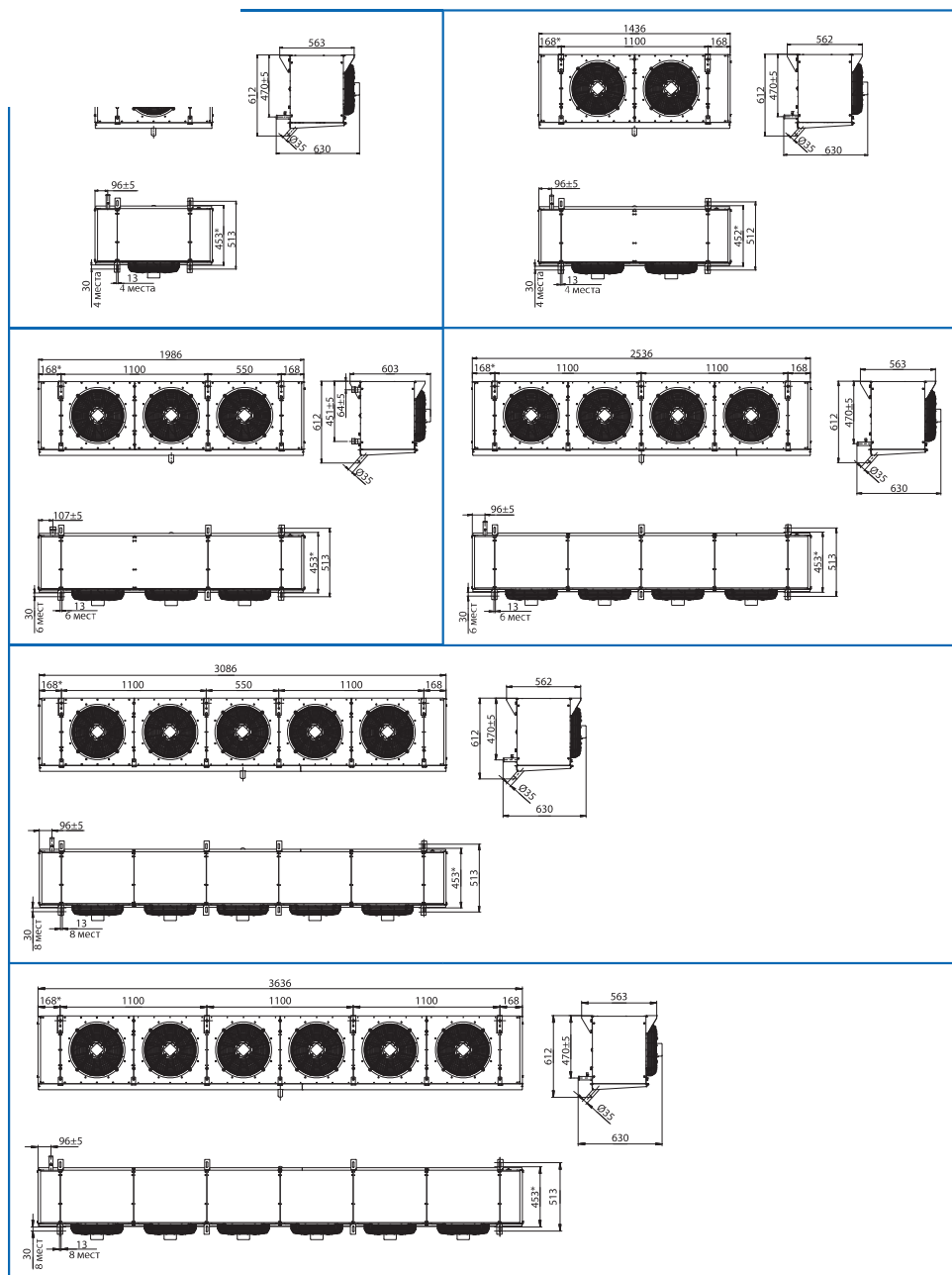
Габаритные и присоединительные размеры UCR.350
